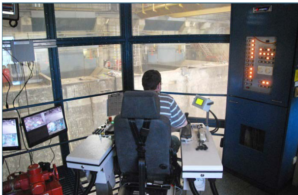
Abb. 30: Kranführer in seiner Kanzel über dem Müllbunker. Im Hintergrund (in Kopfhöhe) erkennt man zwei Trichter zur Aufnahme des Restabfalls für die Verbrennung. Die Öfen liegen jeweils unterhalb davon.
